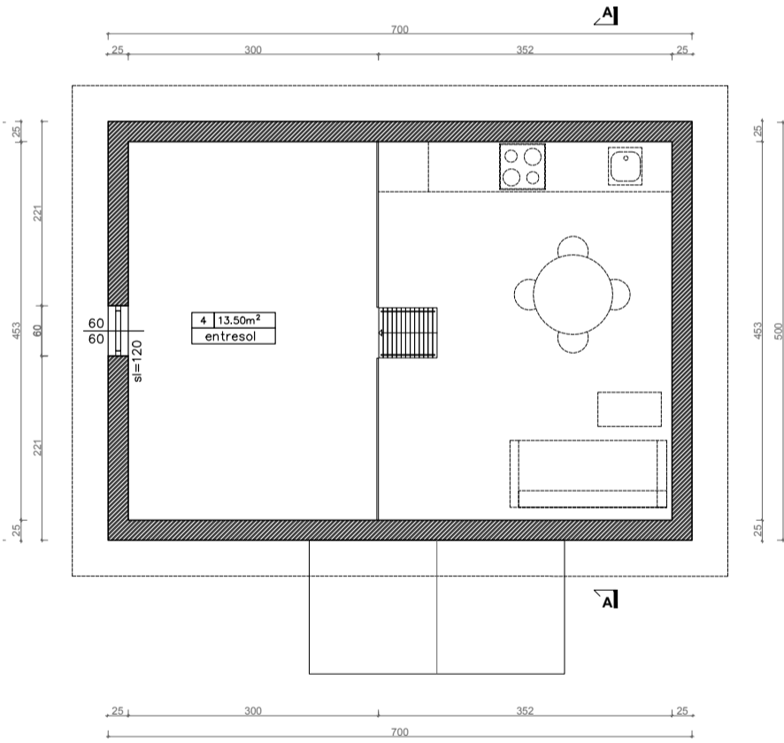
ENTRESOL PLAN
